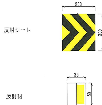
部品図
